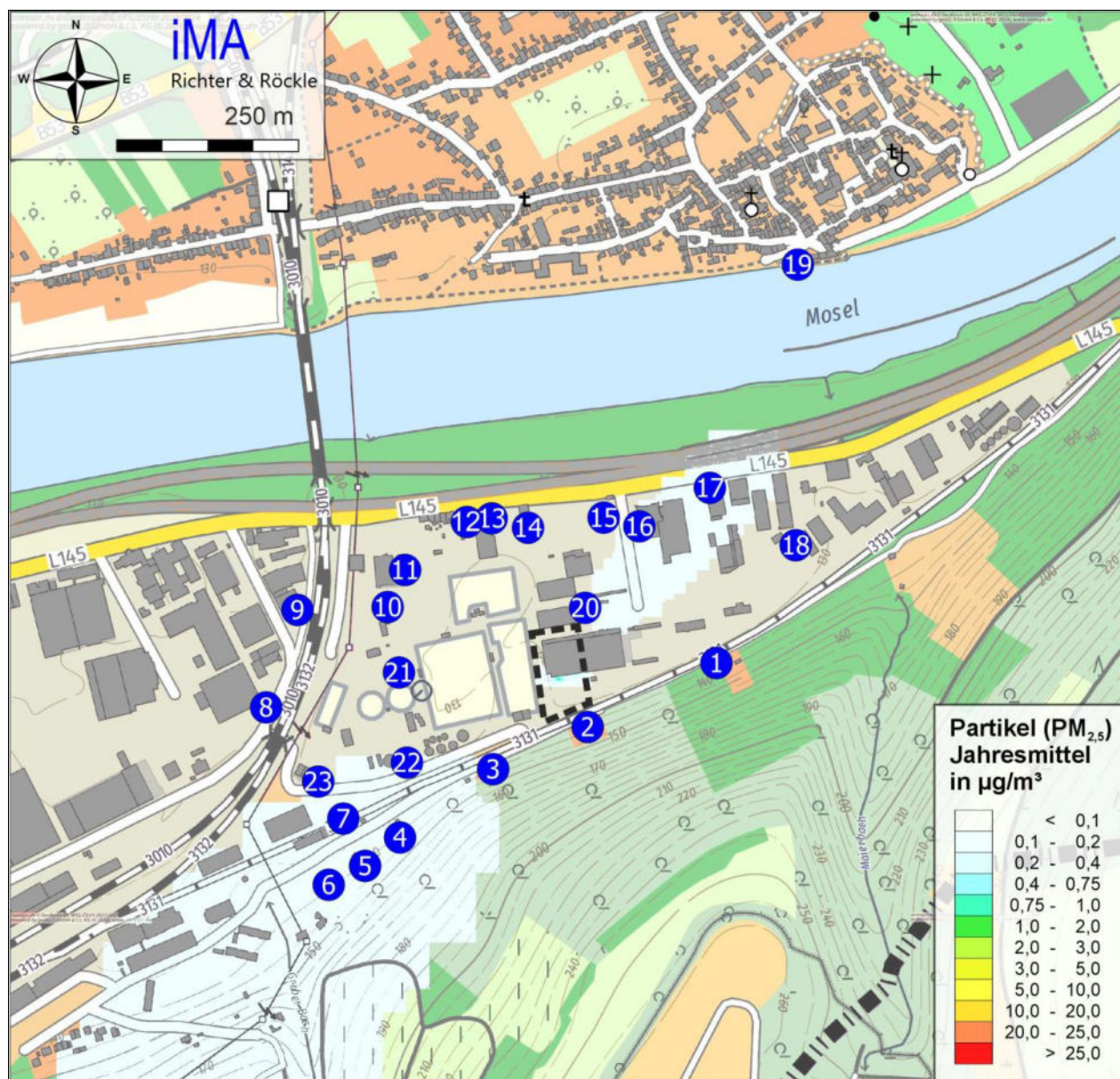
Abbildung A1-2: Gesamtzusatzbelastung der Anlage bzgl. PM 2,5 .
