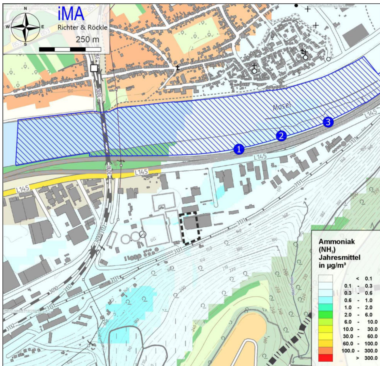
Abbildung A1-8: Gesamtzusatzbelastung der Anlage bzgl. NH 3 : Jahresmittelwerte in µg/m³.
