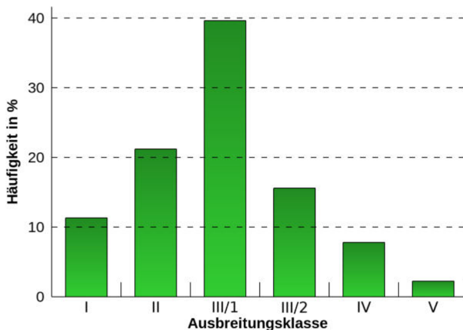
Abbildung 9-4: Häufigkeitsverteilung der Ausbreitungsklassen
